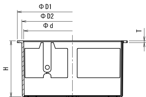
断面 A-A
